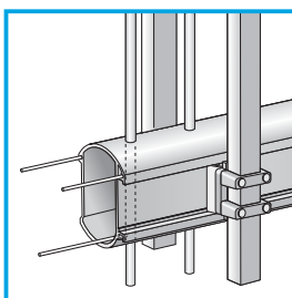
Construction de la lisse par fils de tension
